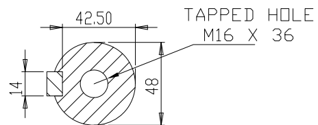
SECTION A-A SCALE 1 : 2
