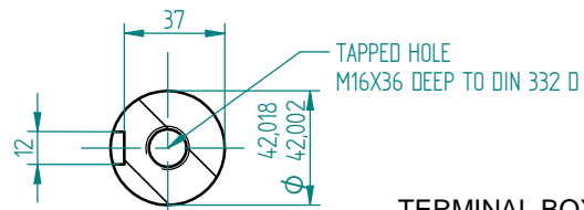
Przekrój A-A 1:2
