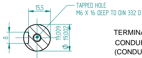
Przekrój A-A 1:1
